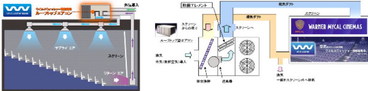
「ルーフトップエアコン組込形 空間清浄システム」構成図
