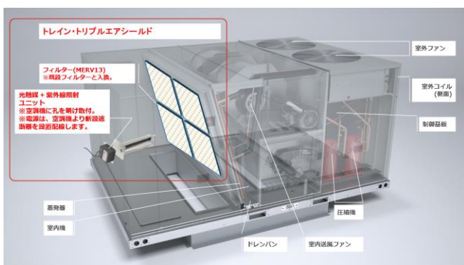
「トレイン・トリプルエアシールド®」本体
