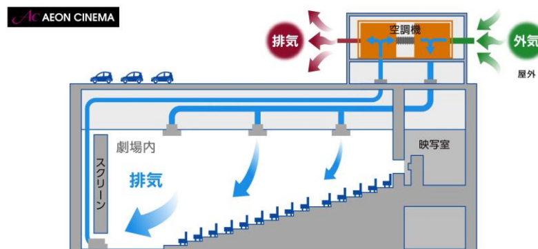
<空調の仕組み>
